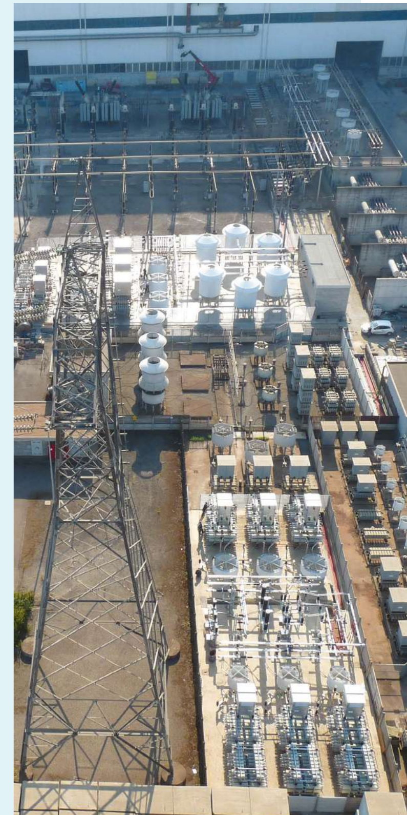
Acciaieria Arvedi - Sistema di rifasamento dinamico 500 MVAR (Cremona) Arvedi Steelworks - 500 MVAR dynamic power factor correction system (Cremona).
